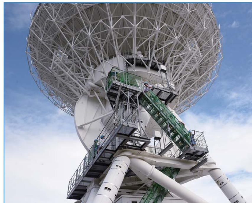
直径20メートルの電波望遠鏡「VERA」のアンテナツアー。下から見ても迫力満点
