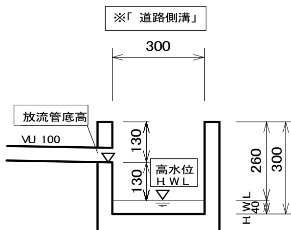
放流先詳細図 S=1:10
