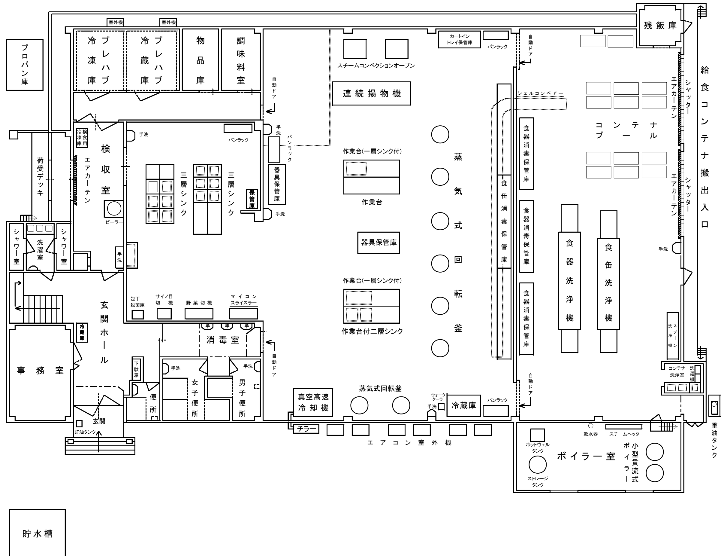
奥州市立江刺学校給食センター施設設備配置図(1F)
