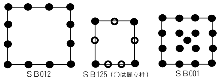
第11図 国見山廃寺跡で発見されている方三間堂
