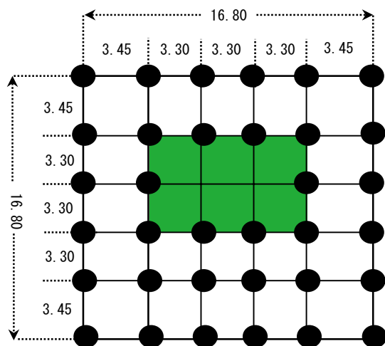
第6図 S B01礎石建物跡の柱配置概念図 (単位m)
