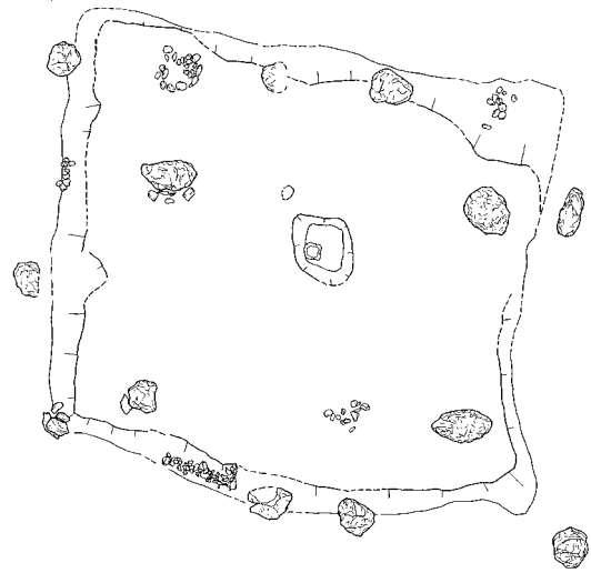
第9図 S B02礎石建物跡平面図（S=1/200）
