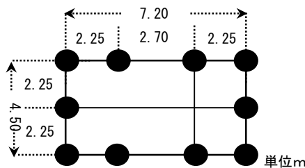
第13図 S B03礎石建物跡柱配置概念図
