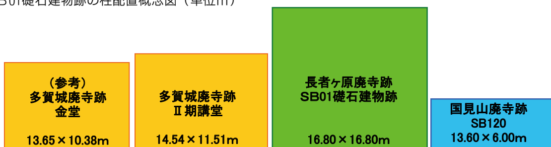
第7図 11世紀の陸奥国の寺院建築規模比較概念図 (S=1/400)
